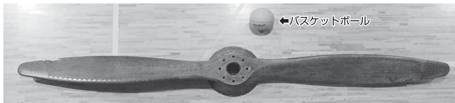
旧日本海軍の九四式水上偵察機に装着されていた木製のプロペラ（長さ3.9m、重さ40kg）前縁を真ちゅうで覆い、強度を高めている。
